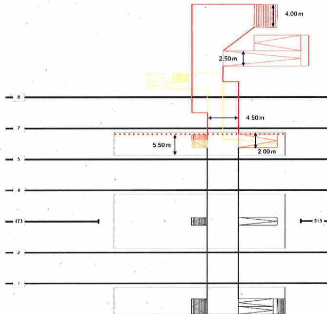
Abbildung 2: schematische Darstellung PU SBB mit provisorischem Anschluss Zustand 2030
