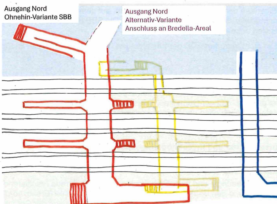
Abbildung 3: Skizze der «Ohnehin-Variante SBB» (rot) sowie der Alternative «Zugang Bredella» (violett) sowie Rückbau der bestehenden PU (gelb)
